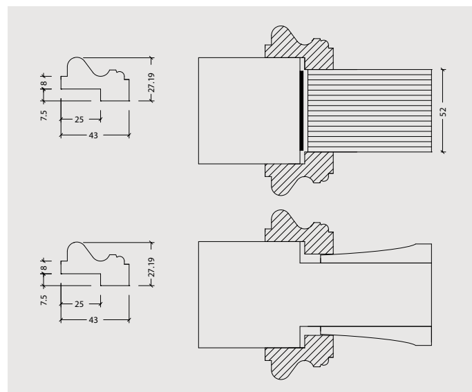
CORNICE SAGOMATA EI 120
