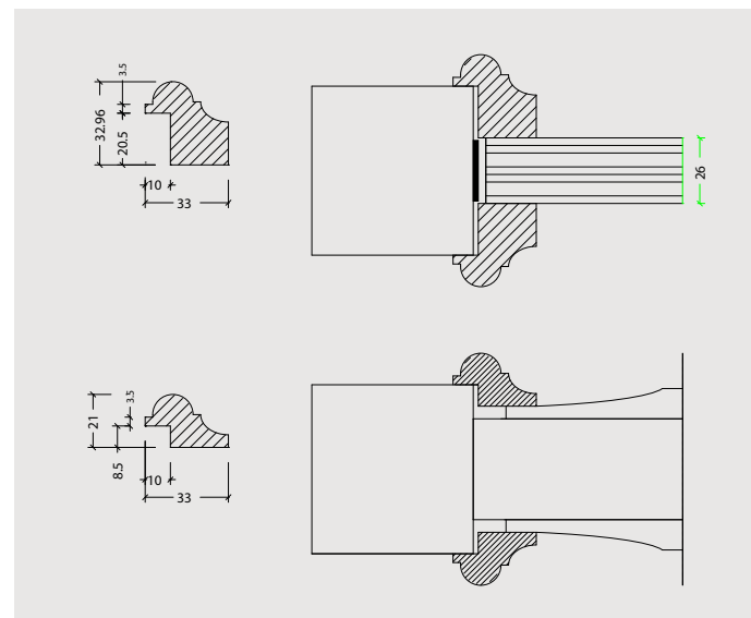
CORNICE SAGOMATA EI 60
